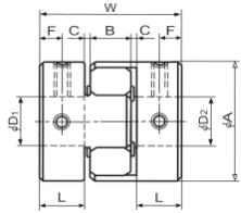
SJC-14 à SJC-30
