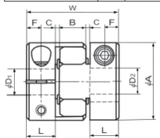
SJC-14C à SJC-30C
