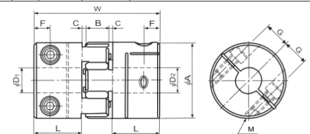
SJC-55C à SJC-80C
