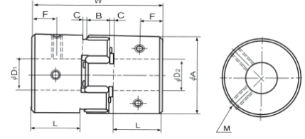
SJC-55 à SJC-80
